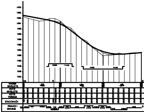
Секундарна унутрашња саобраћајница C-9, од тачке 12 до тачке 8
