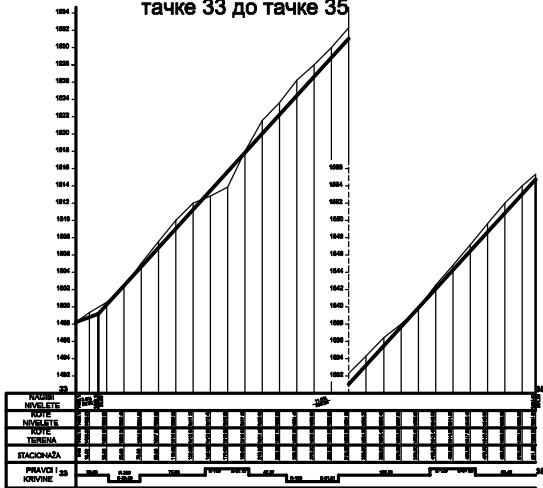
Секундарна унутрашња саобраћајница C-14, од тачке 33 до тачке 35
